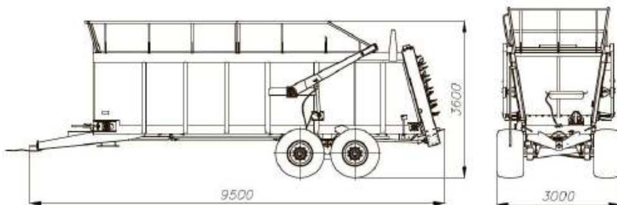
ПОЛУПРИЦЕП МНОГОФУНКЦИОНАЛЬНЫЙ ПМФ-20
