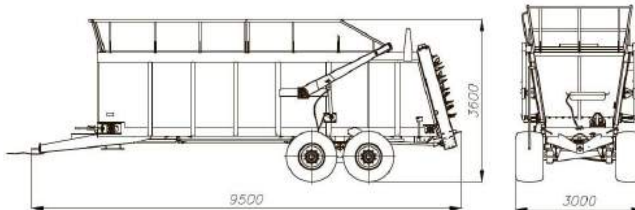
ПОЛУПРИЦЕП МНОГОФУНКЦИОНАЛЬНЫЙ ПМФ-20
